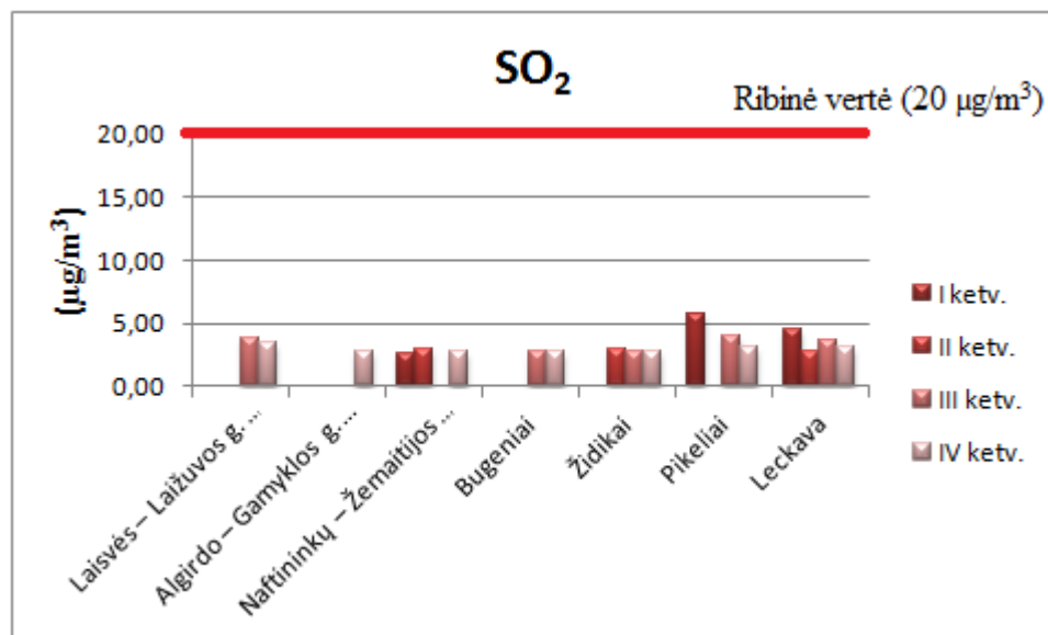
6 pav. SO 2 koncentracijų pasiskirstymas Mažeikių rajone. Ribinė vertė (20 µg/m³).
