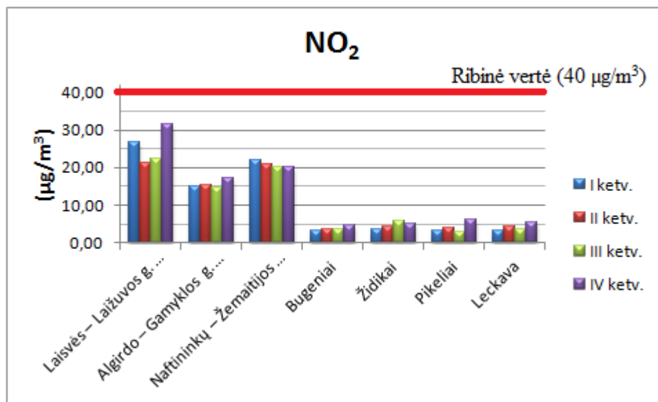
5 pav. NO 2 koncentracijų pasiskirstymas Mažeikių rajone. Ribinė vertė (40 µg/m³).
