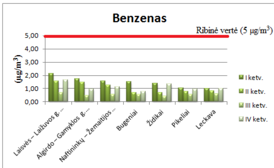
7 pav. Benzeno koncentracijų pasiskirstymai Mažeikių rajone. Ribinė vertė (5 \mu\text{g}/\text{m}^3 ).
